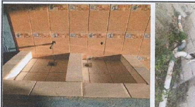
Foto 12: Sustrucción de tubería de red de agua potable, tubería pvc de 1/2 pulga, llave de paso
